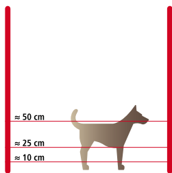
Clôture électrique pour petits chiens Recommandation : hobbysset, tresse
