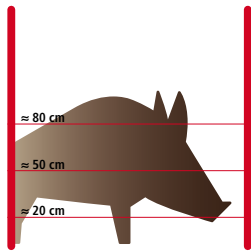
Clôture électrique pour sangliers Recommandation : filet contre gibier AKO, bande de 10 mm, tresse
