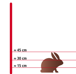
Clôture électrique pour lièvres et lapins Recommandation : filet pour lapins, tresse
