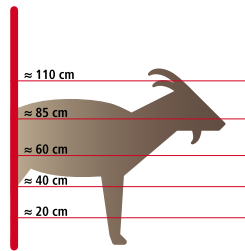
Clôture électrique pour chèvres Recommandation : fils ou tresse
