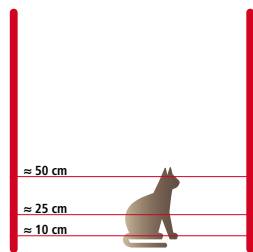
Clôture électrique pour chats Recommandation : hobbysset, tresse
