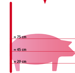
Clôture électrique pour porcs Recommandation : bande de 10 mm, tresse
