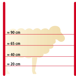
Clôture électrique pour moutons Recommandation : filet, fils ou tresse
