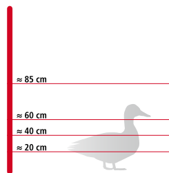
Clôture électrique pour oies Recommandation : filet pour volaille, bande, tresse
