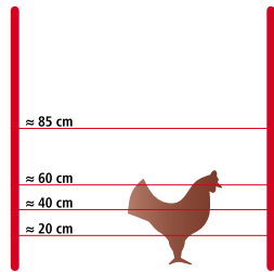
Clôture électrique pour poules Recommandation : filet pour volaille, tresse
