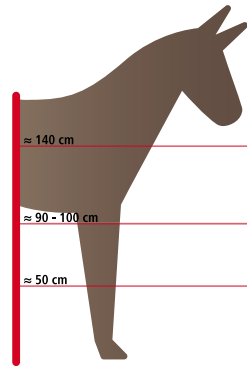
Elektrozaun für Grosspferde Empfehlung: Seil, Breitband bis 40 mm
