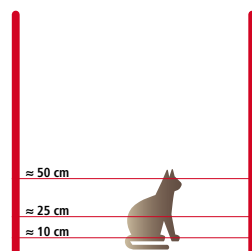
Elektrozaun für Katzen Empfehlung: Hobbyset, Litze
